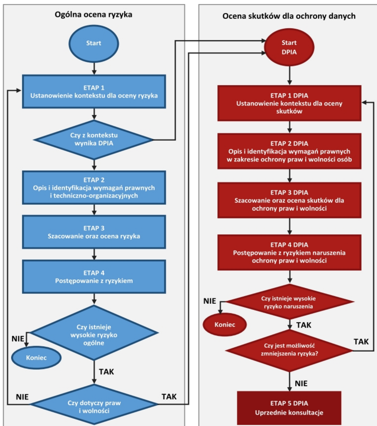
Rysunek 12. Ogólne etapy oceny ryzyka oraz oceny skutków dla ochrony danych.
