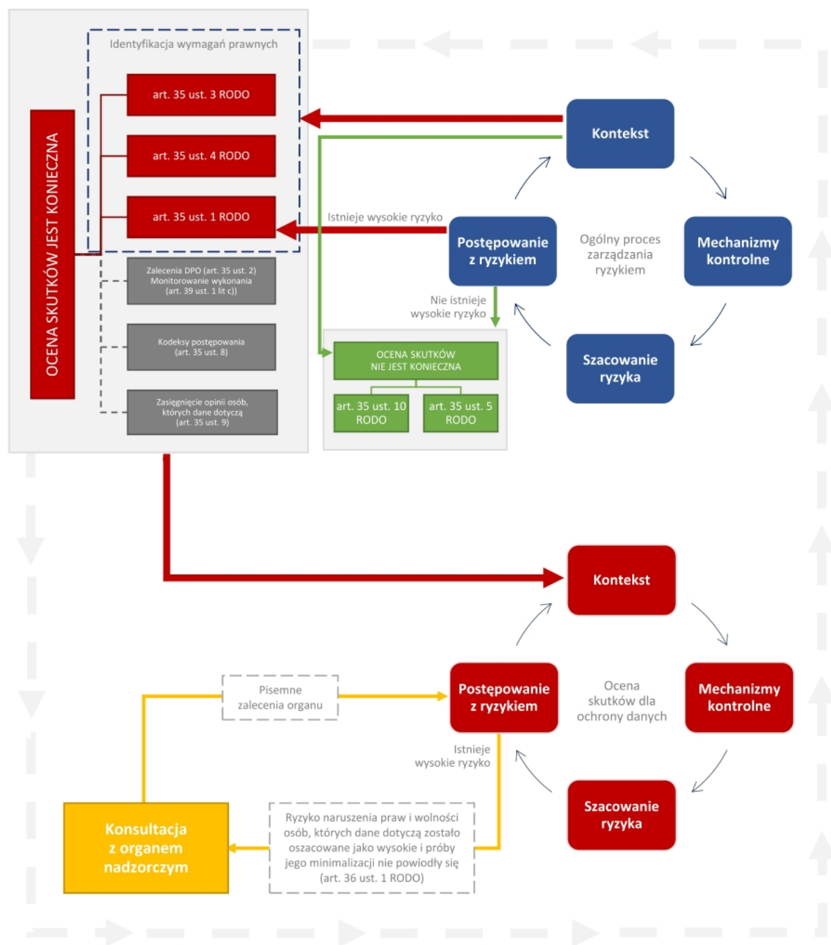
Rysunek 13. Szczegółowe etapy oceny ryzyka oraz oceny skutków dla ochrony danych
